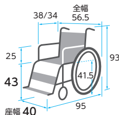
エアリー仕様 (ノーパンクタイヤ)
