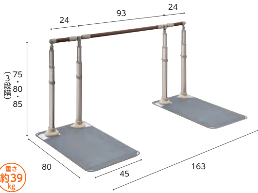
重量 約39kg 片手すり (AT-C-630)
