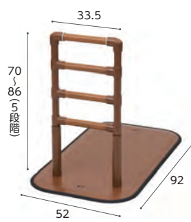
サイドタイプ PJ01-AL 重さ 17 kg
