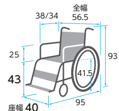
エアリー仕様 (ノーパンクタイヤ)
