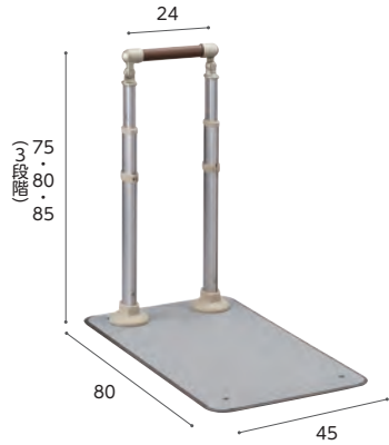
重量 約19kg 片手すり (AT-C-240)
