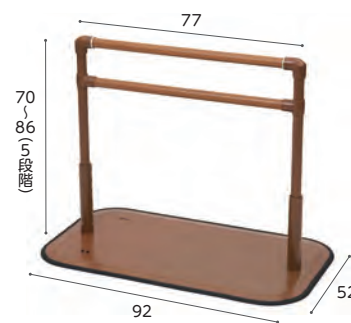
ロングタイプ PJ01-BL 重さ 17.5 kg
