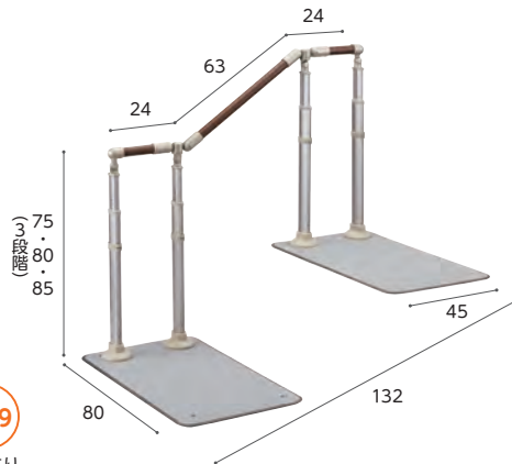
重量 約19kg 片手すり (AT-C-240)
