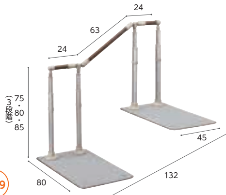
重さ 約19 kg 片手すり (AT-C-240)
