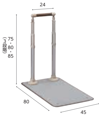
重さ 約19 kg 片手すり (AT-C-240)
