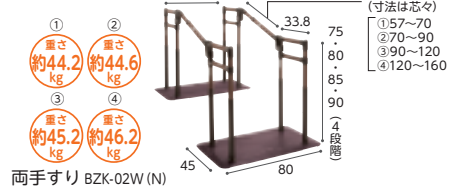
両手すり BZK-02W (N)
