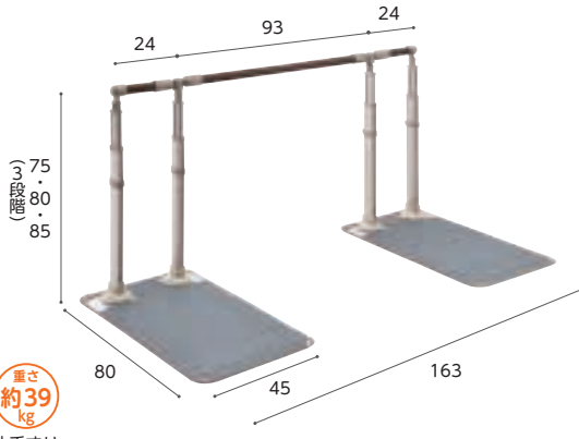
重さ 約39 kg 片手すり (AT-C-630)
